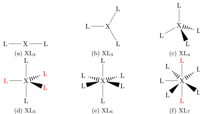
Figure 5: Die verschiedenen Konfigurationen. Rote L zeigen, wo die grossen Domänen eingeführt werden. Punktsymmetrische Geometrien (Linear, Trigonal, Tetraedrisch, Oktaedrisch, Quadratisch Planar) besitzen keine Präferenz.
